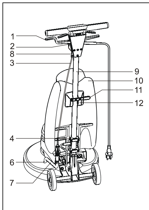
Abb. 8: Flüssigkeitstank montieren
