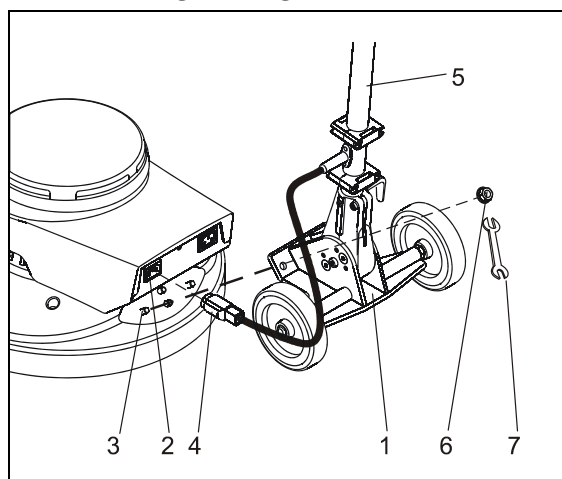
Abb. 5: Führungsstange montieren
