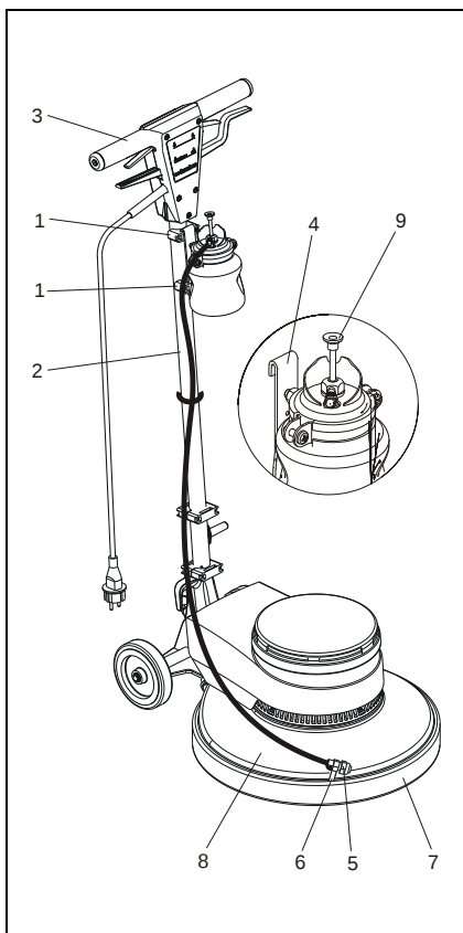
Abb. 7: Sprühgerät montieren
