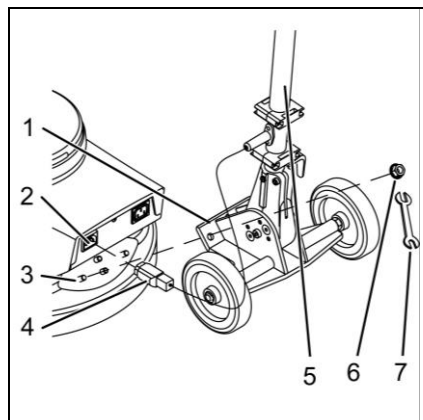
Abb. 5: Führungsstange montieren
