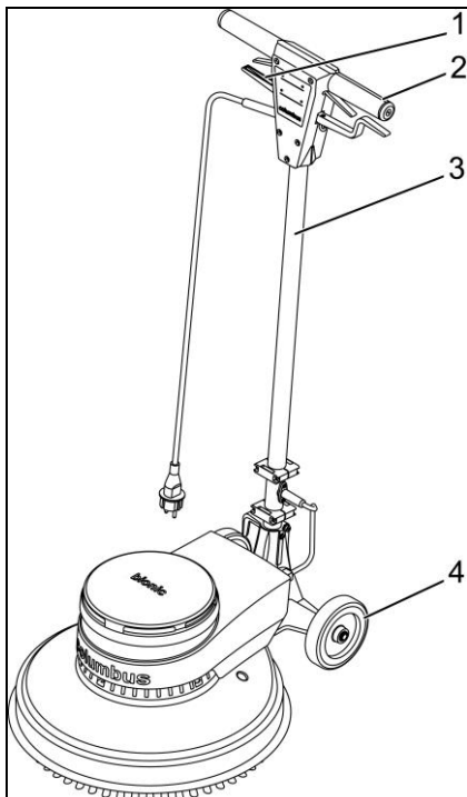
Abb. 13: Führungsstange einstellen
