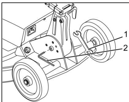
Abb. 14: Drehgelenk einstellen
