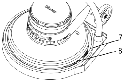
Abb. 11: Absaugring montieren
