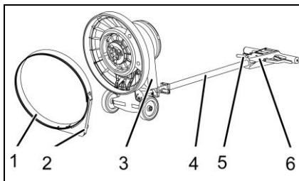
Abb. 10: Sauggerät montieren
