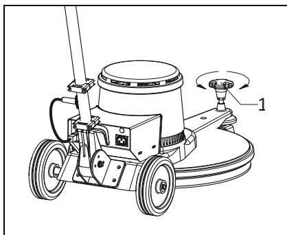
Abb. 12: Arbeitsdruck einstellen
