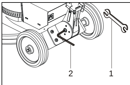
Abb. 11: Drehgelenk einstellen
