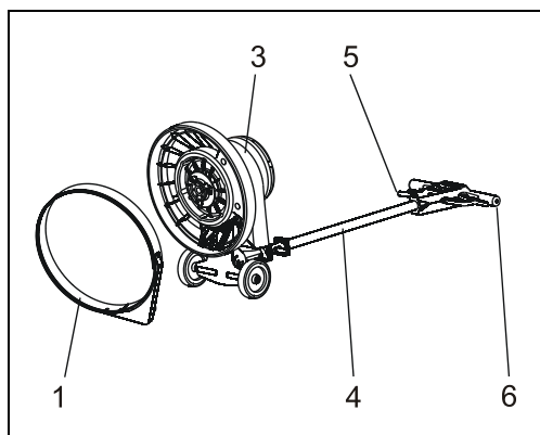
Abb. :: Absaugring montieren
