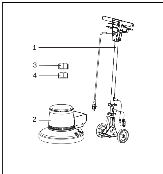
Abb. :: Lieferumfang
