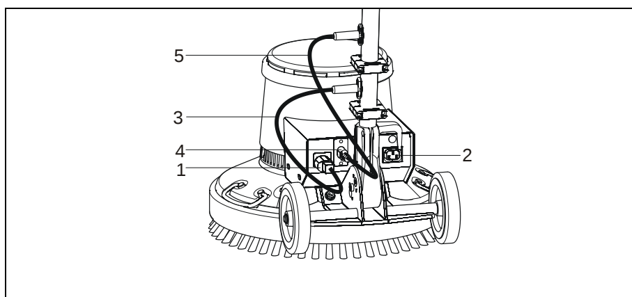
Abb. .: Geräteübersicht/Rückseite
