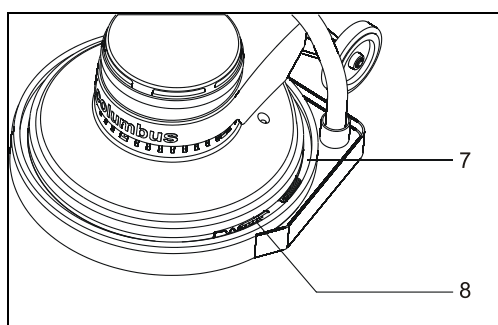
Abb. :: Absaugring montieren
