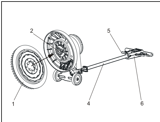
Abb. .: Reinigungswerkzeug manuell einsetzen
