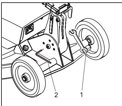
Abb. : Drehgelenk einstellen
