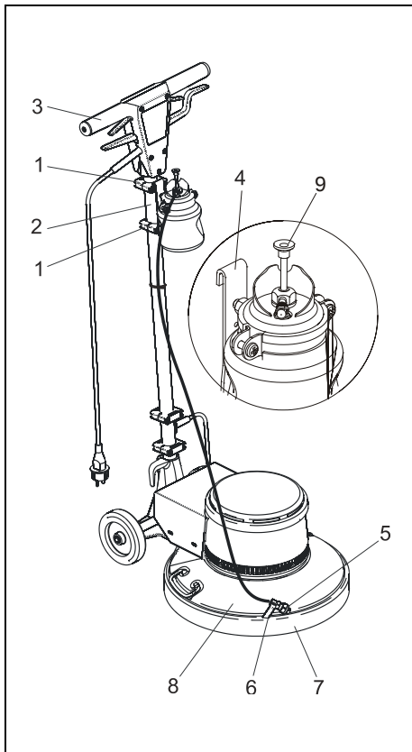
Abb. :: Sprühgerät montieren
