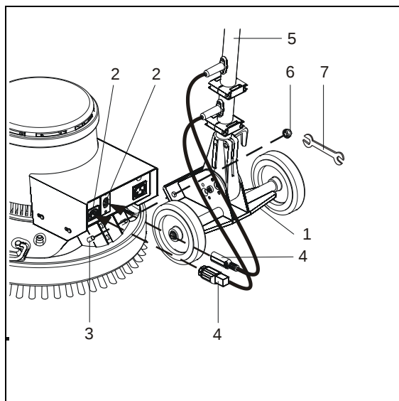
Abb. :: Führungsstange montieren
