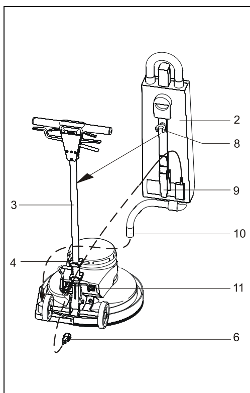
Abb. :: Saugbehälter montieren
