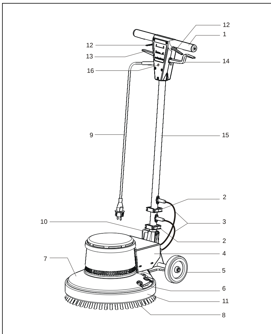
Abb. .: Geräteübersicht
